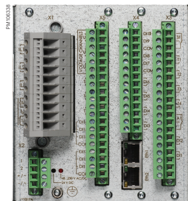
PowerLogic™ P3U30
