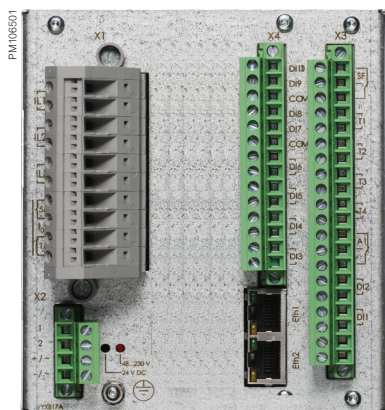
PowerLogic™ P3U20
