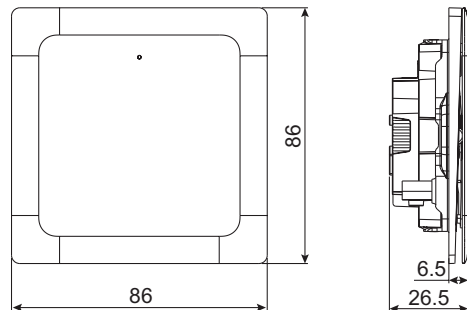
1G Switch
