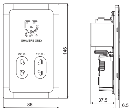
Shaver Sockets
